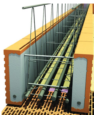
Príklad výstuže prekladu Porotherm KP XL
