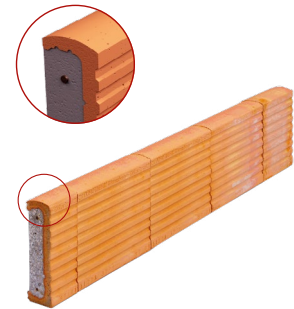
Rozmery prekladu v reze 70 x 238 mm (š x v)
