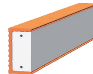
Porotherm KP Vario 100-175 (rozmery v reze: 125 x 238 mm)
