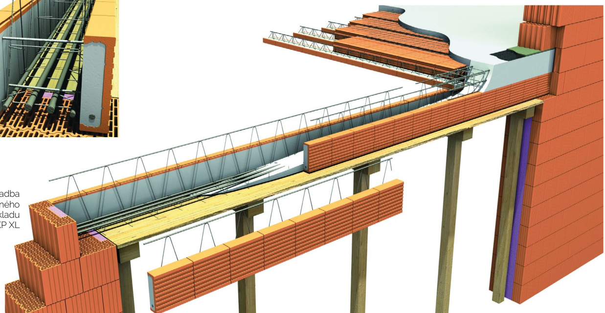
Príklad výstuže prekladu Porotherm KP XL
