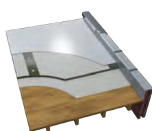
mechanické kotvenie fólie pomocou LRS pásov
